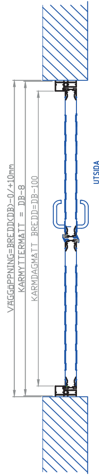
A - A HORIZONTALSEKTION
